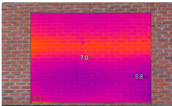
Mise en évidence d'un pont thermique (projet DPE_IITI Noisiel 2013)
