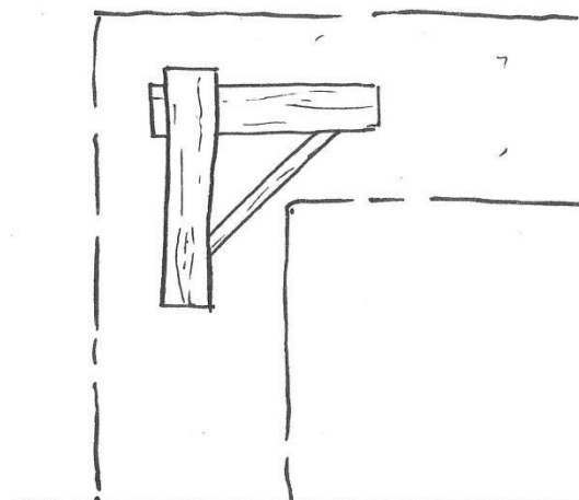
Figure 26: Agrafe* en chêne ou châtaigner
