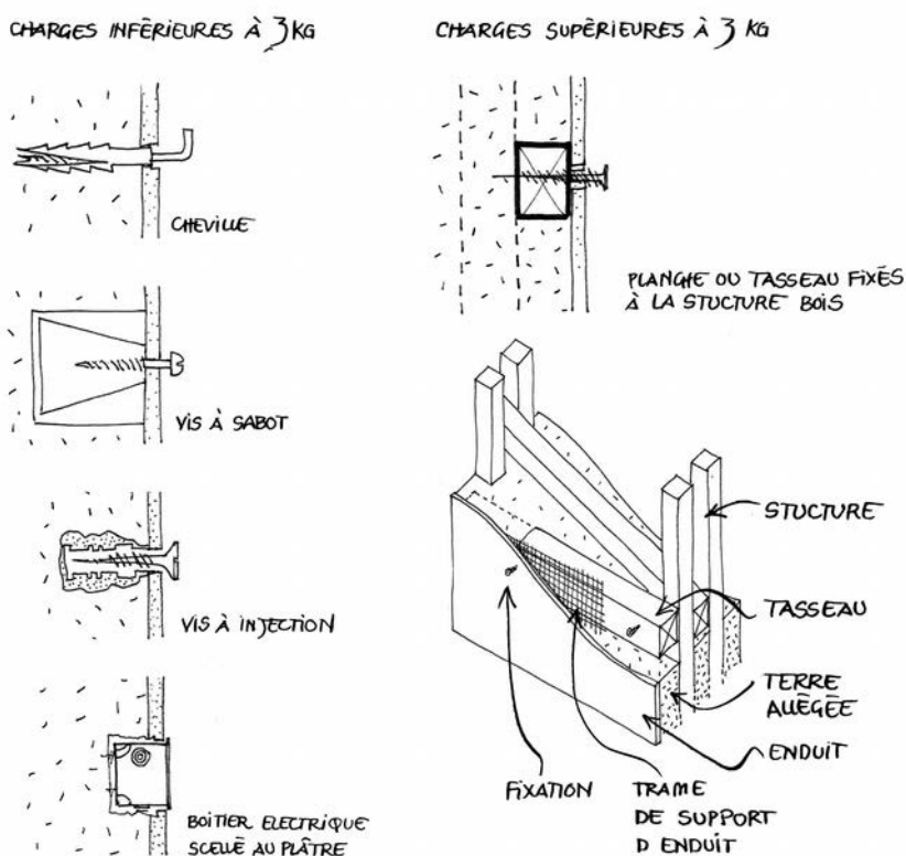
Figure 9: Fixations de charges intérieures
