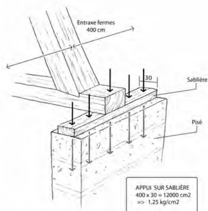
Ferme sur sablière
