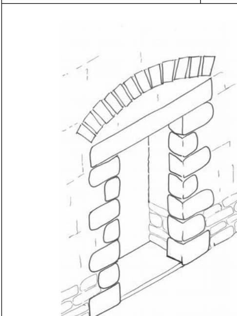
Figure 44: Encadrement en pierres avec arc de décharge*
