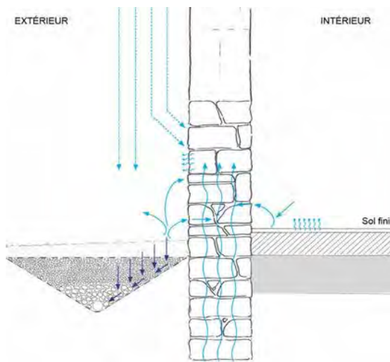
Figure 11: Fondation et soubassement* en pierre, sol en terre enherbée en pente (10%) + drain* enterré
