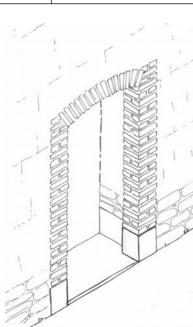
Figure 45: Encadrement en briques
