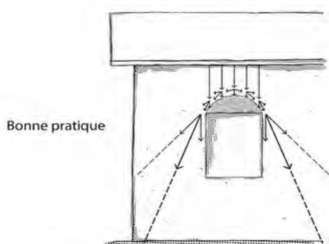
Dessin 10: incidence du report des charges sur les appuis (jambages) d'une ouverture et positionnement aux angles
